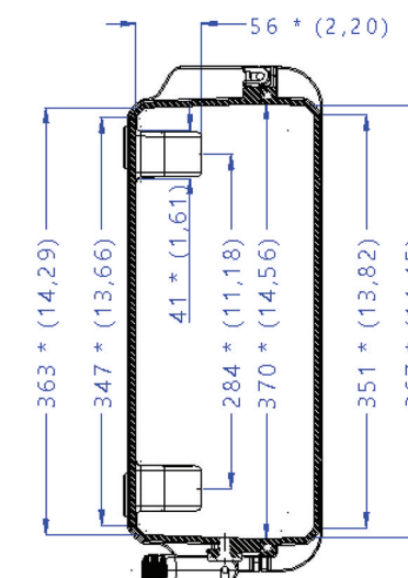
Розріз B-B Section B-B
