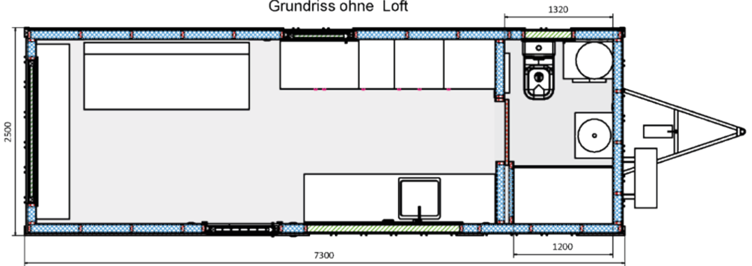
Grundriss ohne Loft
