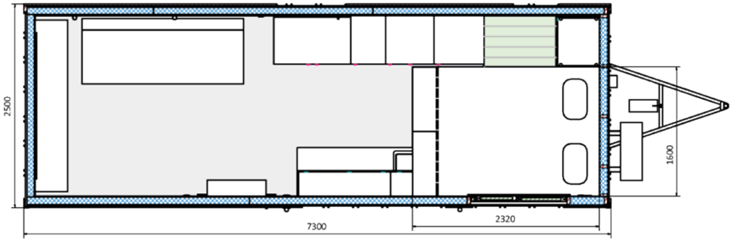
Grundriss ohne Loft
