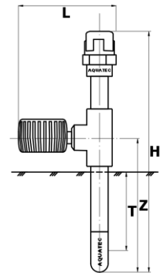
Рисунок 1 Тензіометр AQUATEC іригаційний, серія AQUAMETER PRO, модель TM (міні)
