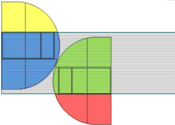
Abbildung 2. Diagramm des Polycarbonatschneidens
