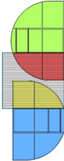
Abbildung 3 - Diagramm des Polycarbonatschneidens an den verbleibenden Teilen der Gewächshausenden
