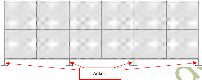
Abbildung 9 - Montage der Anker am Boden
