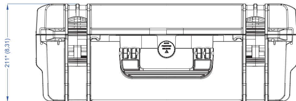
Вид спереду Opening Side
