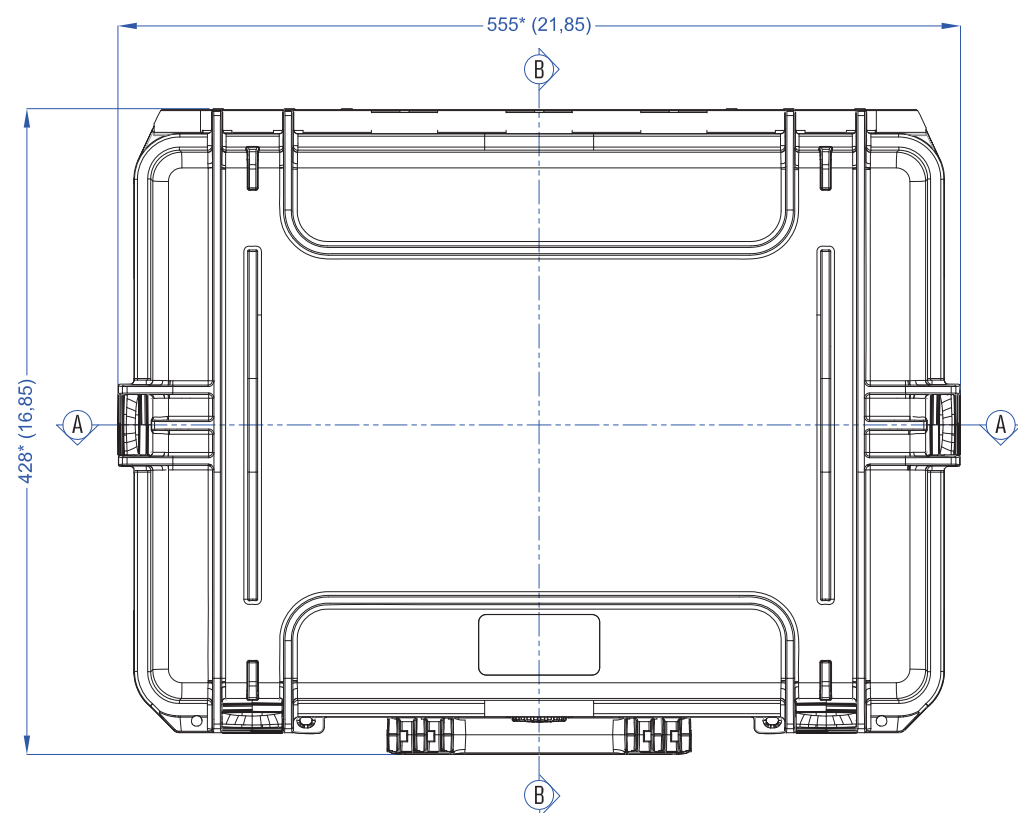
Вид зверху Lid View
