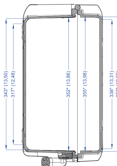
Розріз B-B Section B-B
