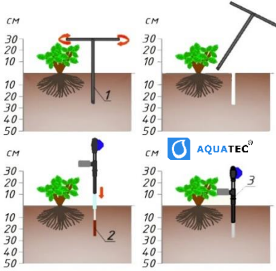
Рисунок 2 Рекомендована схема встановлення тензіометра в ґрунті: 1 – ручний бур; 2 – ґрунтова паста; 3 – тензіометр AQUAMETER PRO, модель Т
