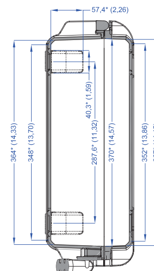
Розріз B-B Section B-B
