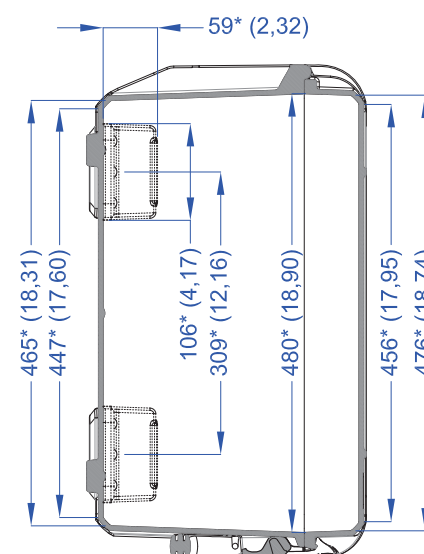
Розріз B-B Section B-B
