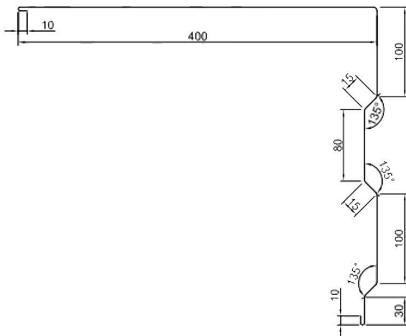
планка покрівельна торцева 2 ППТ-2-775
