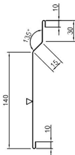
планка відводу цокольна 4 ПВЦ-4-205
