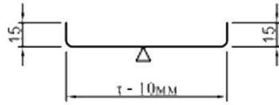
планка замикання панелі 1 ПЗП-1
