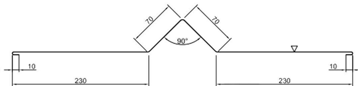
планка покрівельного деформаційного шва зовнішня ПДШЗ-620
