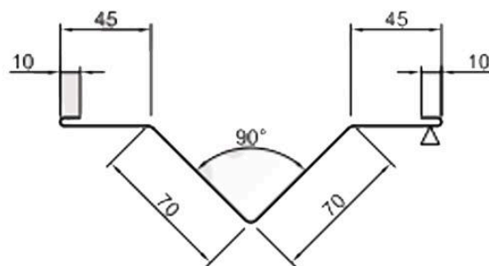
планка покрівельного деформаційного шва внутрішня ПДШВ-250
