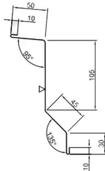
планка упирання фасаду в стіну ПУФС-250
