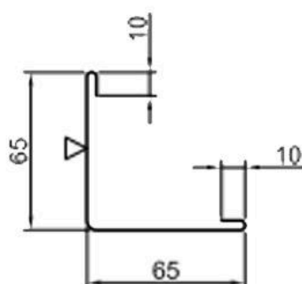
планка вигнутого кута фасаду 5 ПВКФ-5-150
