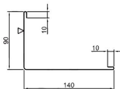
планка вигнутого кута фасаду 4 ПВКФ-4-250
