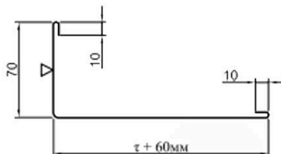
планка вигнутого кута фасаду 3 ПВКФ-3
