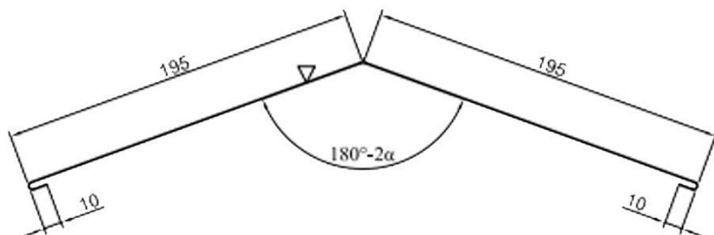
планка конькова зовнішня ПКЗ-410
