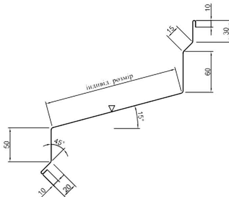
планка відводу цокольна 2 ПВЦ-2
