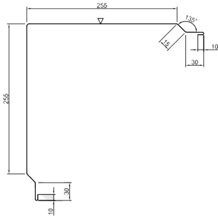
планка вигнутого кута фасаду 1 ПВКФ-1-620
