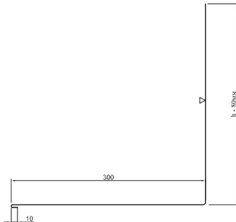
планка примикання покрівлі до парапету ППП
