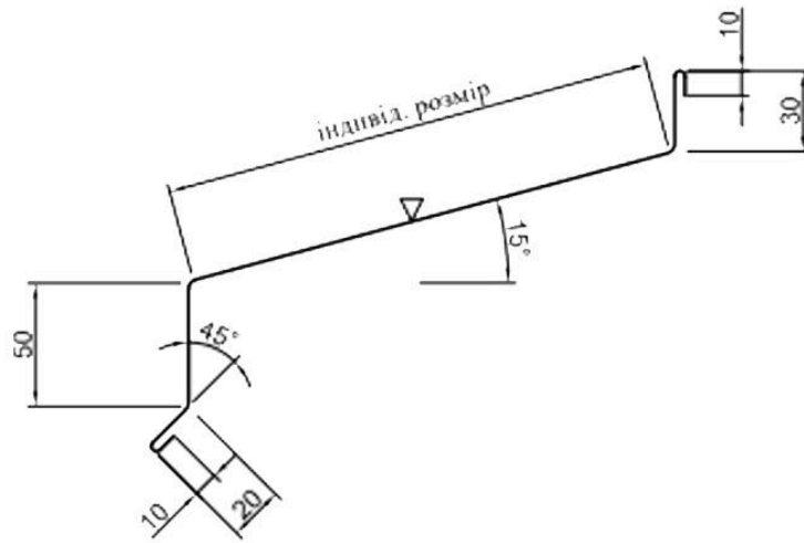
планка відводу цокольна 1 ПВЦ-1
