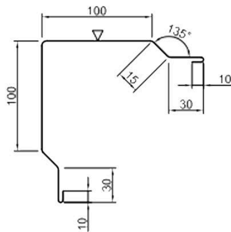
планка вигнутого кута фасаду 2 ПВКФ-2-310
