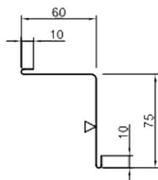
планка примикання покрівля-стіна ПППС-155
