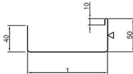
планка замикання панелі 3 ПЗП-3
