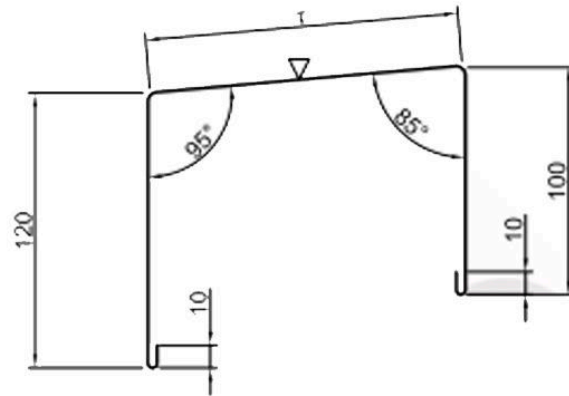
планка парапетна ПП
