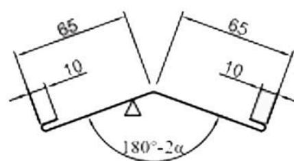
планка конькова внутрішня ПКВ-150
