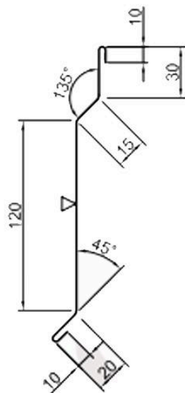
планка відводу цокольна 3 ПВЦ-3-205
