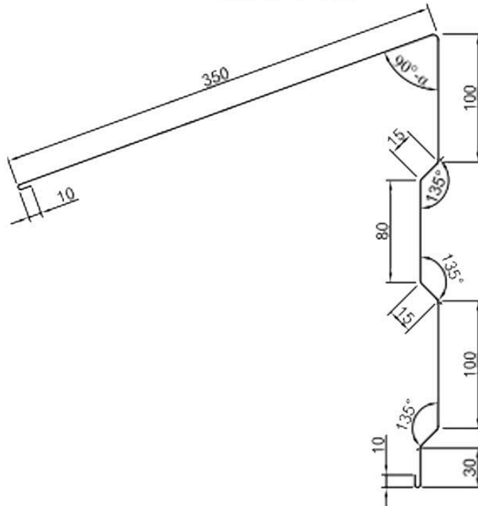
планка гребеню односкатного 2 ПГО-2-725
