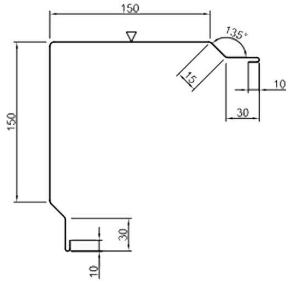
планка вигнутого кута фасаду 6 ПВКФ-6-410
