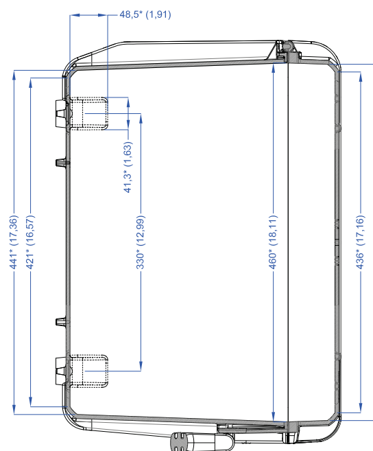
Розріз B-B Section B-B
