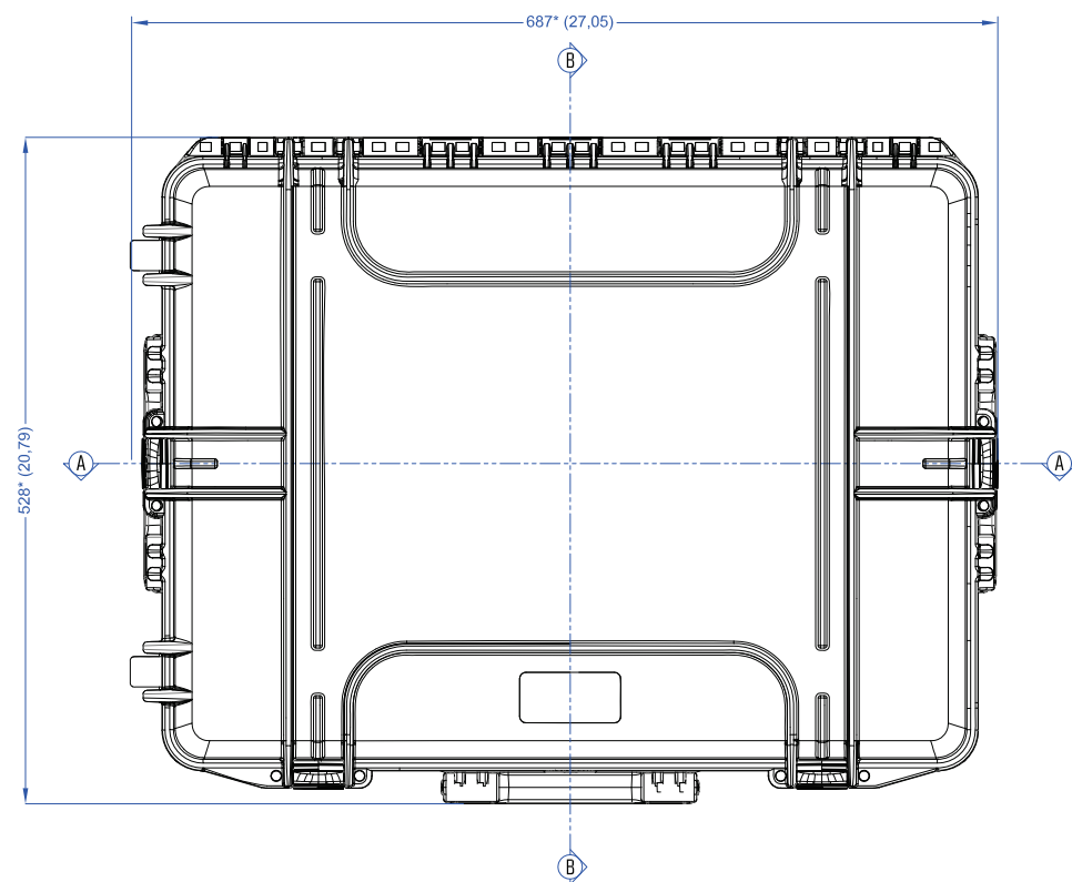
Вид зверху Lid View
