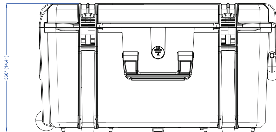
Вид спереду Opening Side
