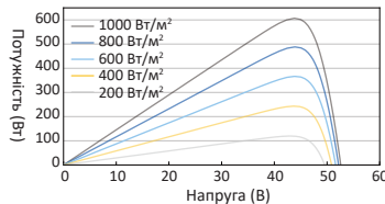
Крива «потужність-напруга» JAM72D40-590/LB
