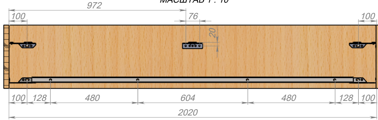
РОЗРІЗ А-А МАСШТАБ 1 : 10
