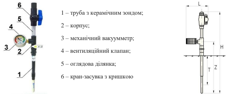
Рисунок 1 Тензіометр AQUATEC іригаційний, серія AQUAMETER PRO, модель T GL
