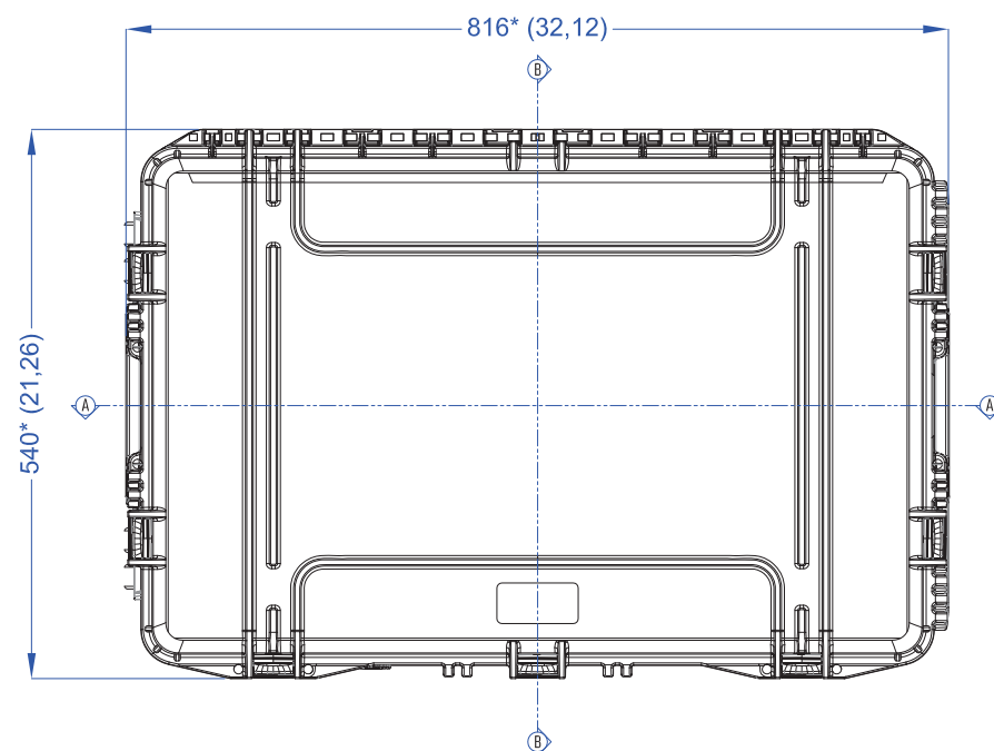
Вид зверху Lid View
