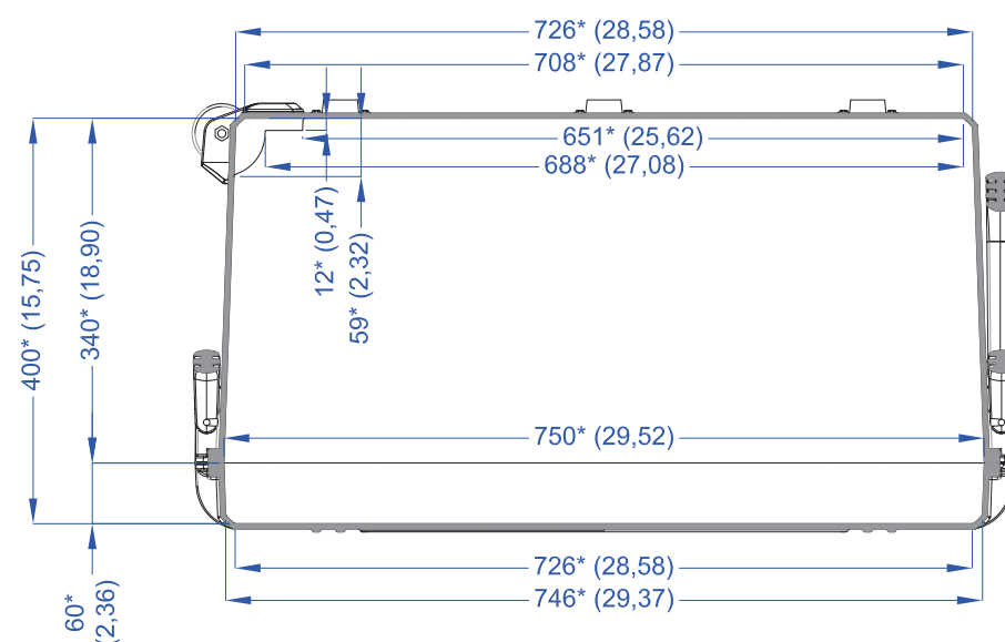
Розріз A-A Section A-A
