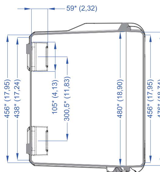
Вид збоку (з права) Side View
