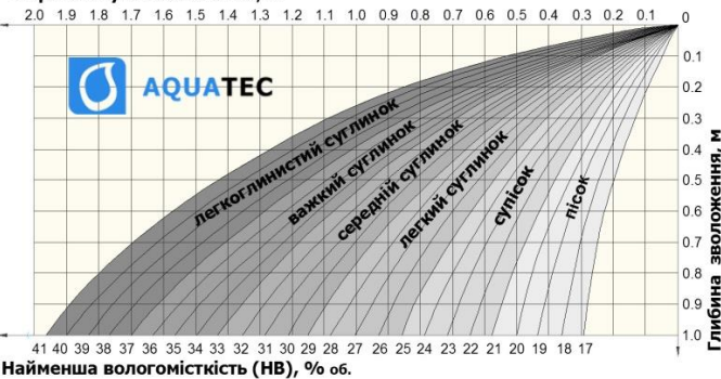
Рисунок 3 Графіки для визначення ширини смуги зволоження за заданою глибиною зволоження для ґрунтів з різними значеннями НВ
