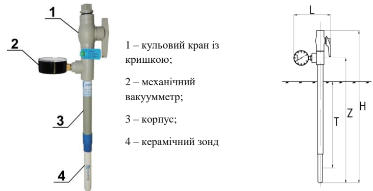
Рисунок 1 Тензіометр вологості ґрунту AQUATEC , серія AQUAMETER ECO , модель T
